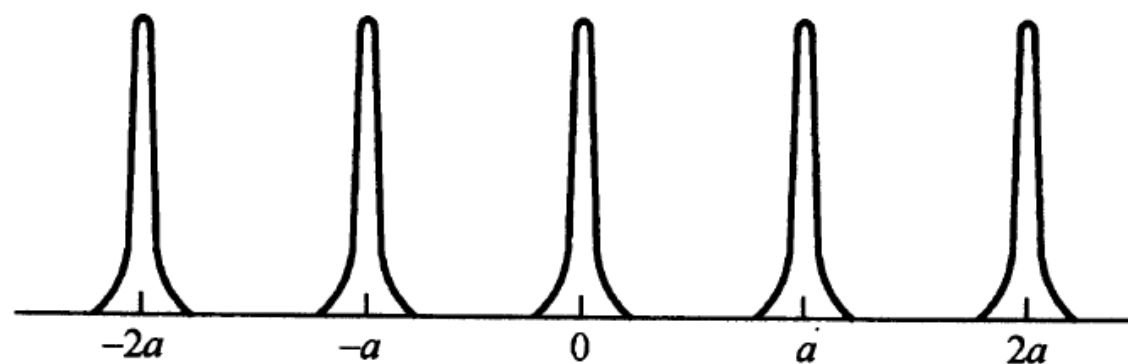
图 3.33 Dirac 梳
