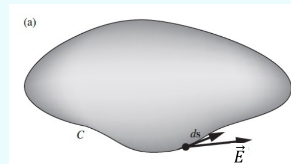
線積分
