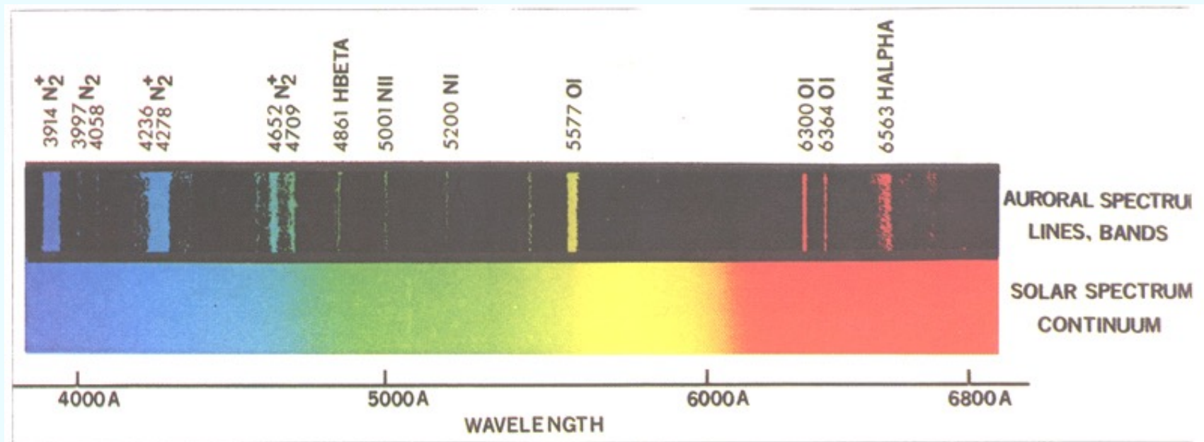
圖5. 極光光譜。
