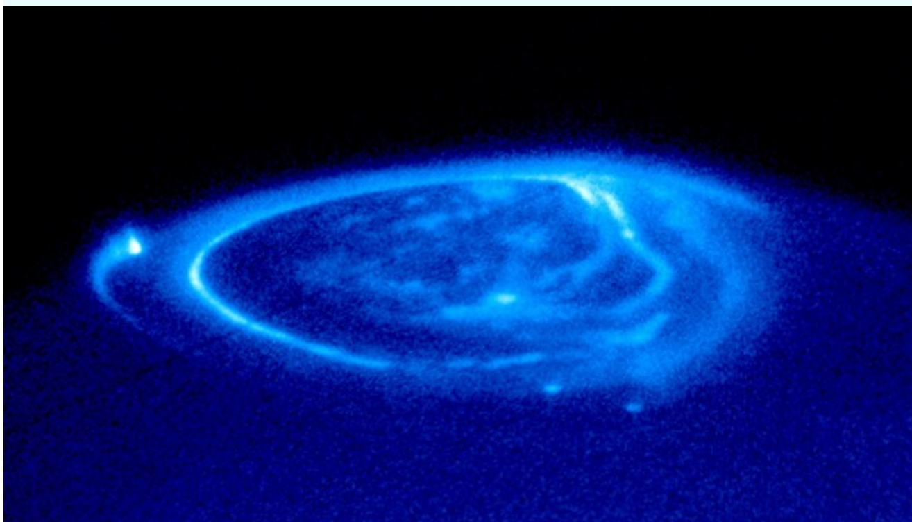
木星
