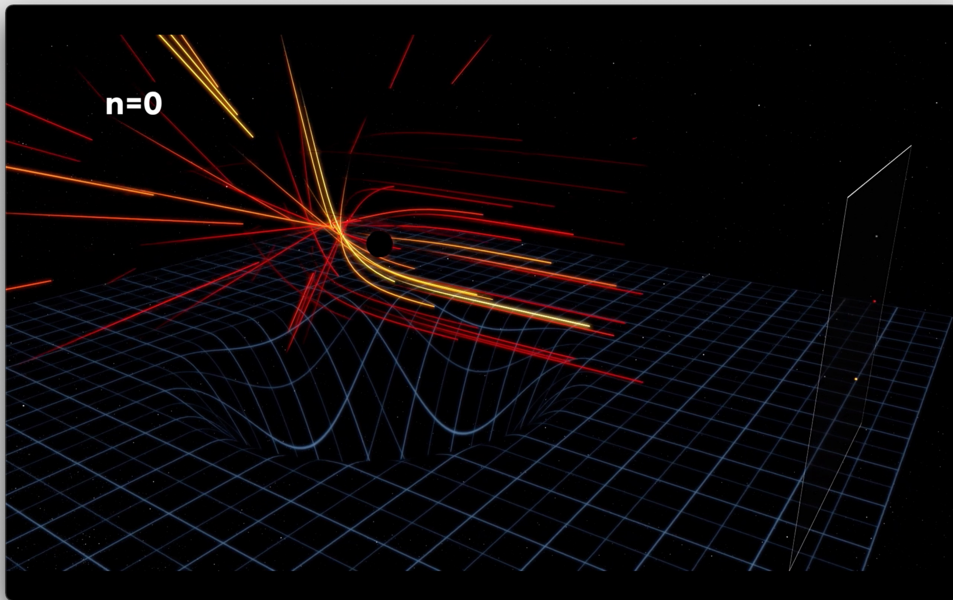
光的測地線
